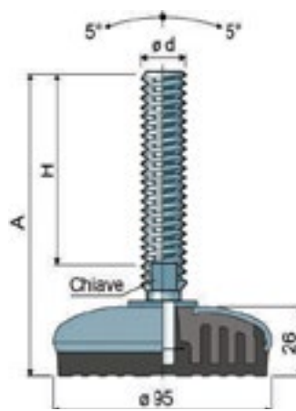
PIEDE ORIENTABILE D.95 Art. 496 Swivel Foot D.95 Art. 496
