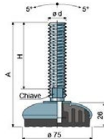
PIEDE ORIENTABILE D.75 Art. 498 Swivel Foot D.75 Art. 498
